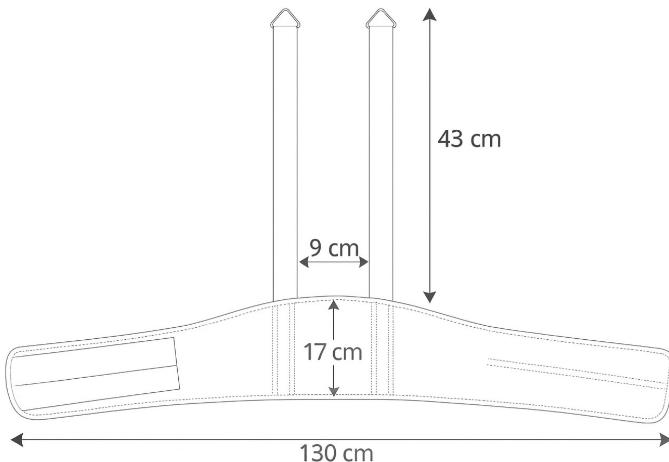
Wymiary pasa KC-13 (skaj) - schemat.
